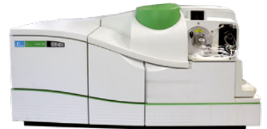
▶ SPEKTROSKOPIE
